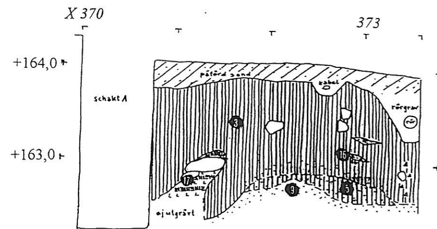
Profil G x370/ y519,5 - x 373,3/ y 519,5 skala 1:40
