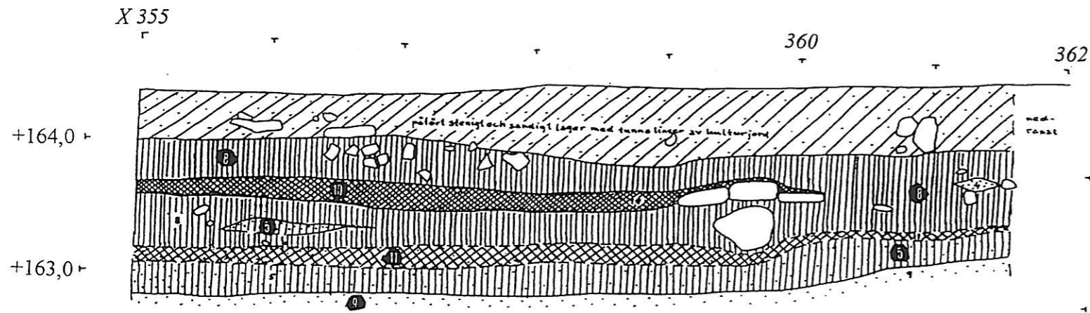
Profil D x355/ y527 - x362/ 527,5 skala 1:40
